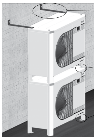
Εικόνα 2: Στοιβαξή
