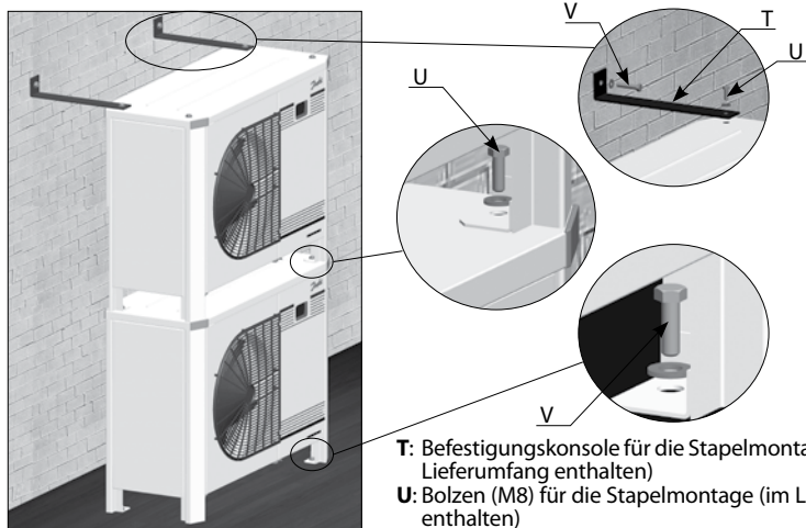
Bild 2: Stapelmontage
