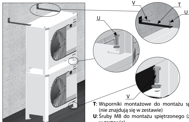
Rysunek 2: Montaż ściętrzony
