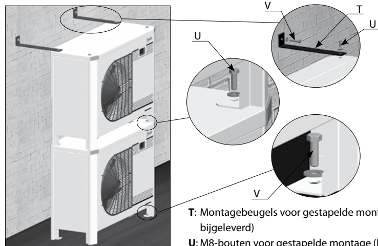
Afbbeelding 2: Gestapelde montage
