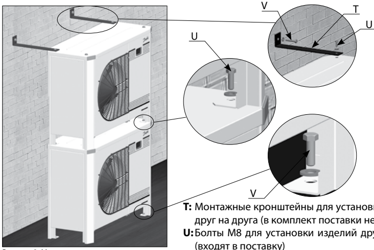
Рисунок 2: Многоуровневое размещение
