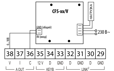
FH аналоговый выход 0...10 В с внешним модулем CFS-xx/V
