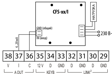
FH аналоговый выход 4...20 мА с внешним модулем CFS-xx/I
