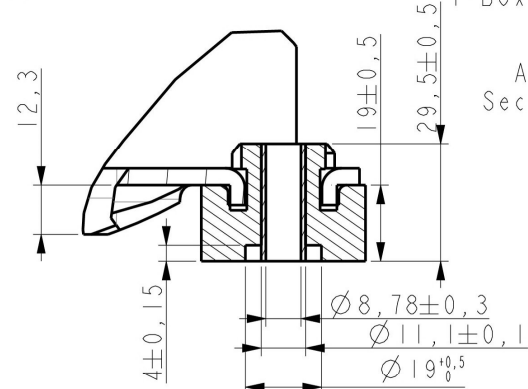
细节 压缩机底脚 Detail Foot 比例 0,750
