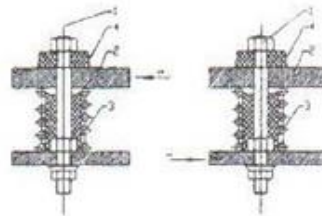
Жесткий монтаж
